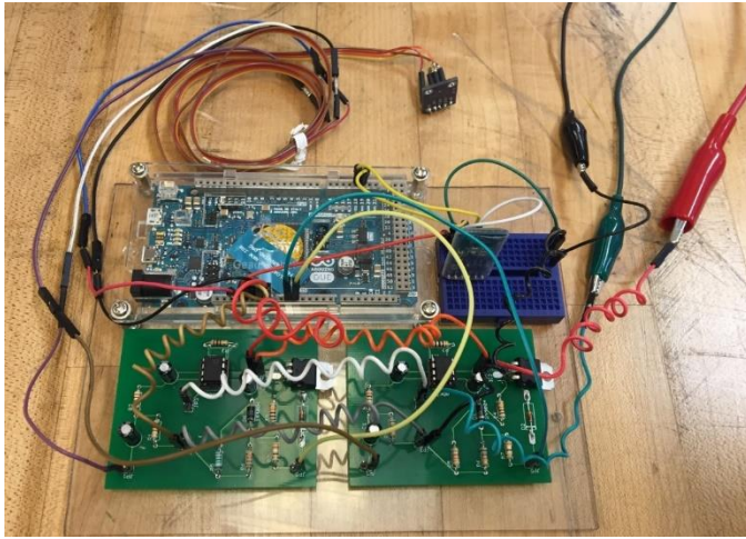
Fig. 8 Actual circuit
